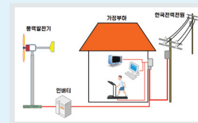
< 풍력시스템 구성도 >
